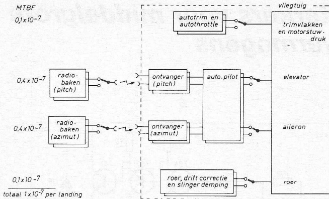
Fig. 16. De MTBF (tijd tussen twee fouten) per groep.
