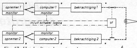
Fig. 17a. Het duplicated monitored systeem uit de VC10 en BAC 1-11.
