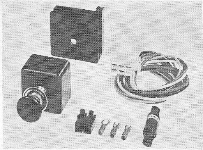
Afb. 1. Een compact gebouwde intervalschakelaar van Bosch met bevestigings- en aansluitmaterialen.
