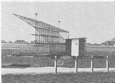
Afb. 10 Koerslijn-zender (Localizer) antenne voor CAT III op Schiphol.
