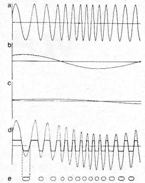
Fig. 10. De signalen voor helderheid (a), kleurinformatie (b) en geluid (c) worden gecombineerd in een amplitudeverhouding 20 : 4 : 1. Het rechthoekige impulssignaal met twee constante amplitude-niveaus en variabele afstanden wordt verkregen door een symmetrisch begrenzingsproces van de som van de afzonderlijke frequenties.
