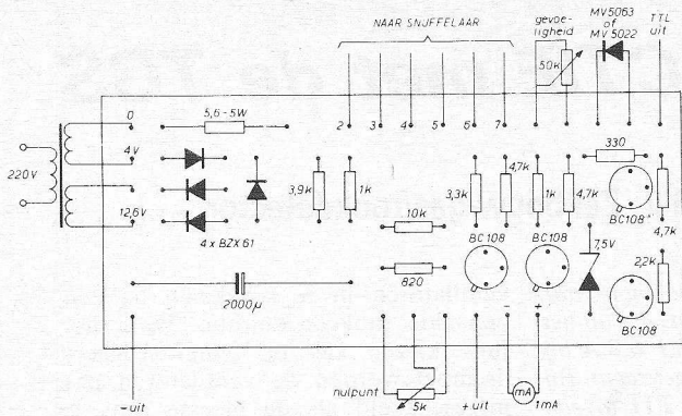
Fig. 2a en b. Printje voor de schakeling van fig. 1.
