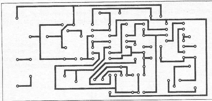
Fig. 4.b. Printje van de uitbreiding.
