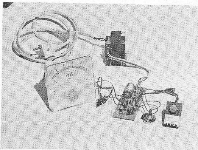
Afb. 1. Proefopstelling van de gas/rook detector.
