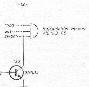
Fig. 3. Uitbreiding van de signalering met visuele voorwaarschuiving en zoemer-alarm.
