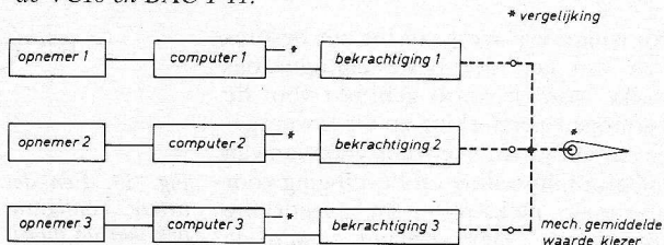
Fig. 17b. Het triplex systeem uit de Boeing 747B. B
