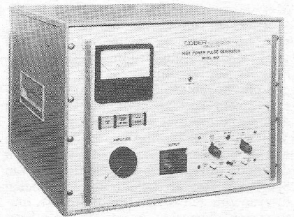
combinaties van spanning en stroom, binnen het maximale vermogen kunnen worden gerealiseerd. Het uitgangscircuit is zwevende t.o.v. aarde met 5 kV DC. De impuls-kwaliteit wordt aangegeven door de scherpe stijgtijd van 20 ns en afvaltijd van 30 ns. Inl.: A. D. Auriema-Europe, Ouderkerk a/d Amstel-Brussel.
