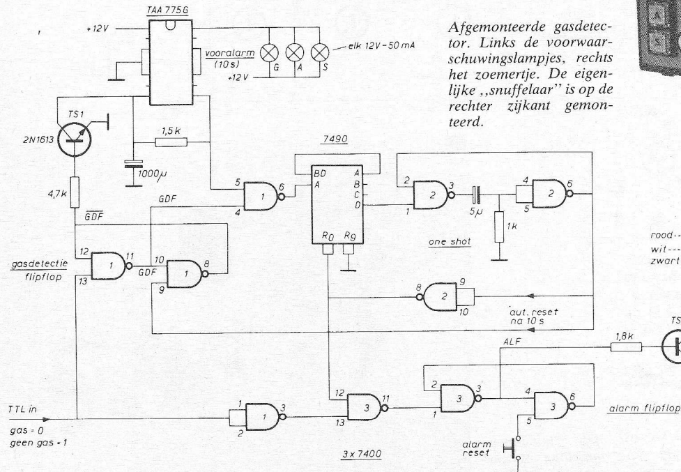
Fig. 3. Uitbreiding van de signalering met visuele voorwaarschuiving en zoemer-alarm.
