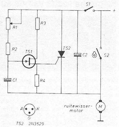
Fig. 7. Volelektronische intervaluutomaat. (Tek. ontleend aan: „Uw auto en de elektronica“.)
