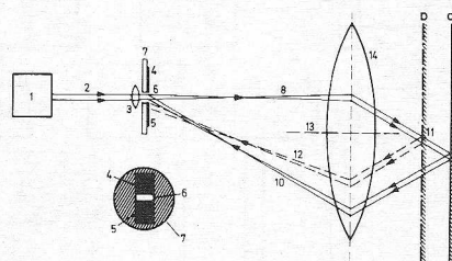
Fig. 8. Schematische voorstelling van een optisch systeem voor het verkrijgen van een regelspanning voor het automatische focuseringsysteem.
