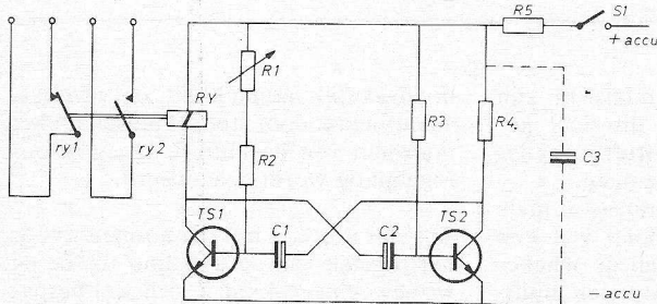
Fig. 8. Intervaluutomaat met multivibratorschakeling. (Tek. ontleend aan: „Uw auto en de elektronica“.)
