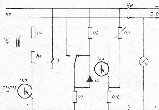
Fig. 4. Elektronische controleschakeling voor de richtingaanwijzers (links).
