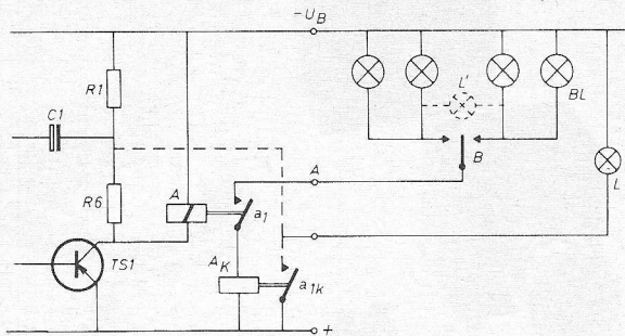
Fig. 3. Controle op de goede werking van de richtingaanwijzers is uitermate belangrijk voor de verkeersveiligheid. Schakeling met een hulprelais, dat alleen voldoende wordt bekrachtigd indien alle lampen van een groep branden.
