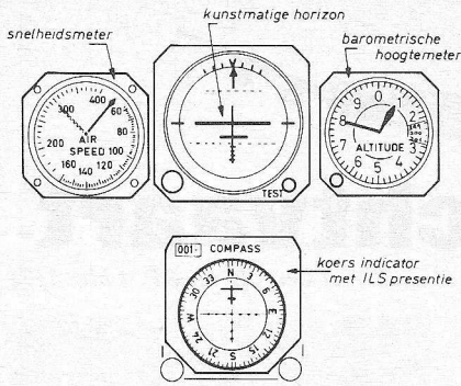
Fig. 13 Opstelling van de belangrijkste vlieg-indicatoren.
