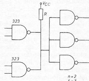
Fig. 9. Voorbeeld van de berekening van de maximale waarde van een collectorweerstand.
