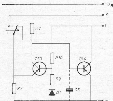
Fig. 4. Elektronische controleschakeling voor de richtingaanwijzers (links).
