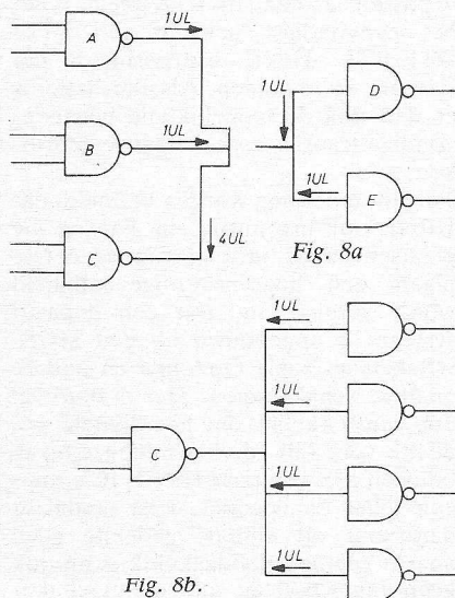
Fig. 8. In beide configuraties wordt poort C belast met 4 UL.
