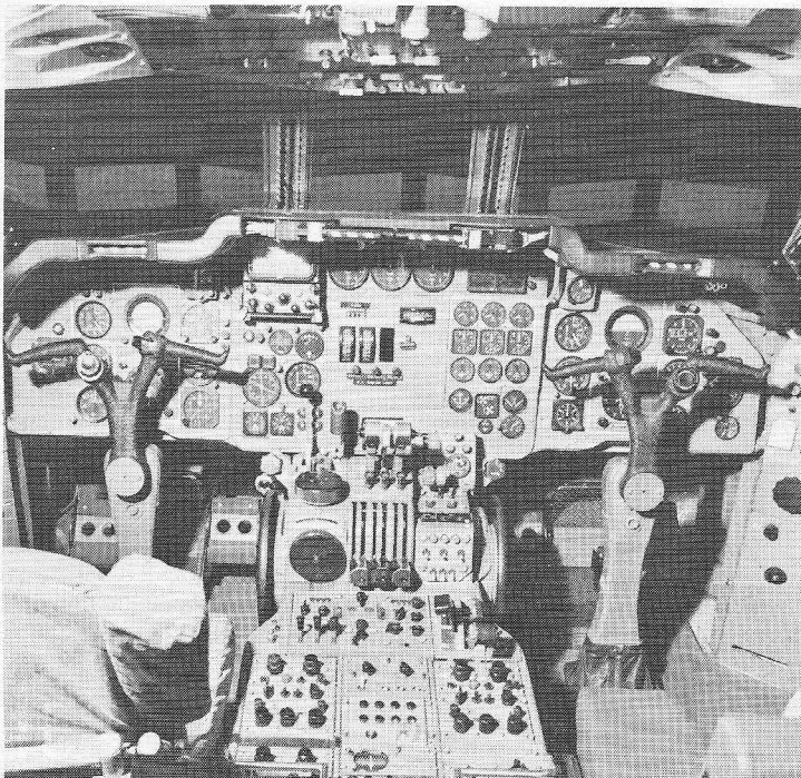
Afb. 15 Deel van de Trident cockpit. In het midden, direct onder de drie gas-handles, het bedieningspaneel van afb. 14.
