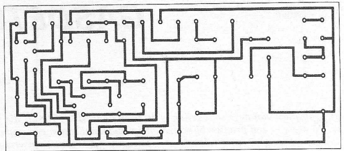
Fig. 2a en b. Printje voor de schakeling van fig. 1.
