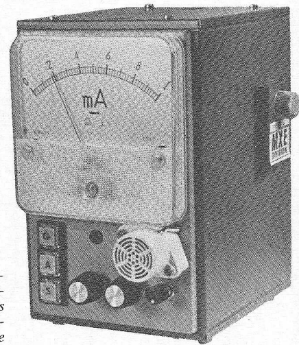
Afgemonteerde gasdetector. Links de voorwaarschuivingslampjes, rechts het zoemertje. De eigenlijke „snuffelaar” is op de rechter zijkant gemonteerd.
