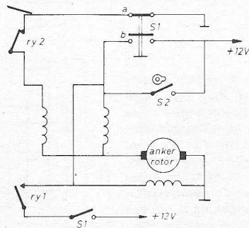
Fig. 10. Schakeling van een ruitwissermotor met veld- en remwikkelingen, alsmede de ingetekende relaiscontacten Ry1 en Ry2. (Tek. ontleend aan: „Uw auto en de elektronica“).
