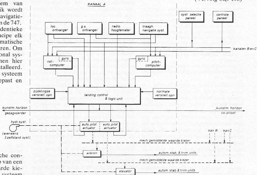
Fig. 18. Een van de drie kanalen uit het vliegregelsysteem van de 747B.
